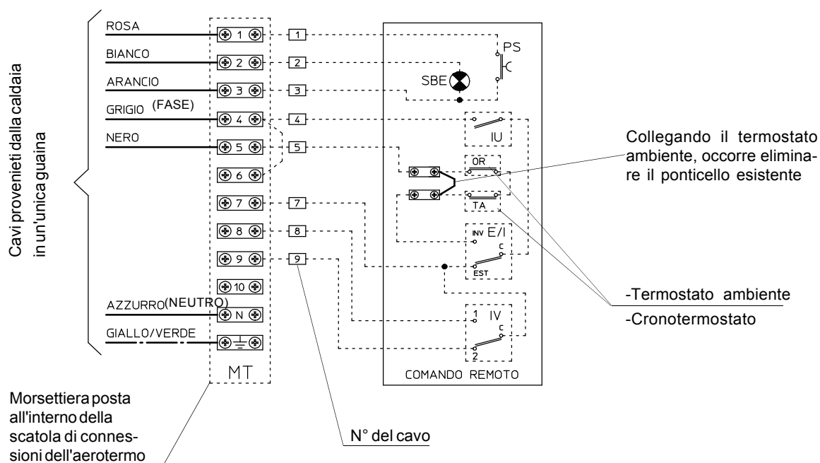
Fig. 8 (HC0042 C2 032) Collegamenti caldaia/unità interna
