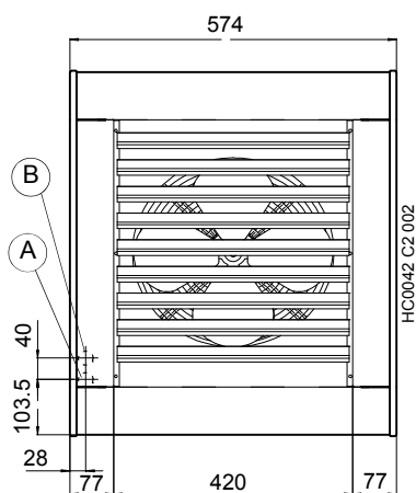
Vista frontale unità 16 kW
