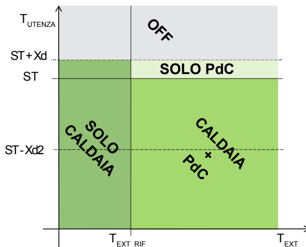
Regolazione invernale con temperatura T_{UTENZA} crescente
