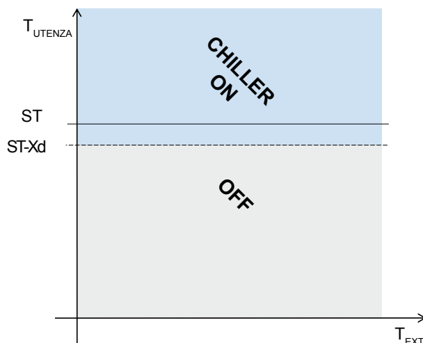
Regolazione estiva con temperatura T_{UTENZA} crescente
