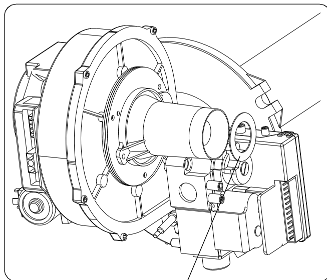
Diaframma aria G2.350 per PL043 - Øi 28 per PL054 - Øi 28 per PL072 - Øi 29
