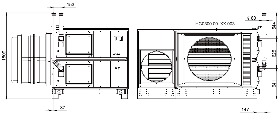
Modello: AH160 / AH210 con scarico fumi SINGOLO
