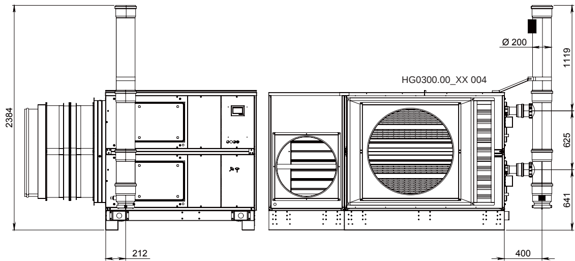
Modello: AH160 / AH210 con scarico fumi COLLETTIVO
