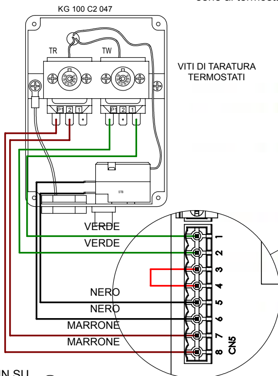
VITI DI TARATURA TERMOSTATI
