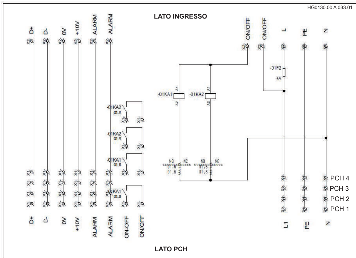
Schema elettrico della morsettiere di interfaccia
