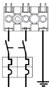
Collegamento 230 V
