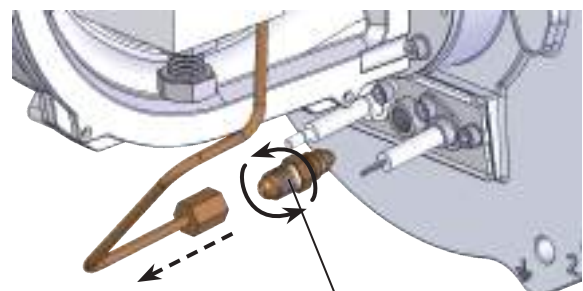
Ugello pilota
