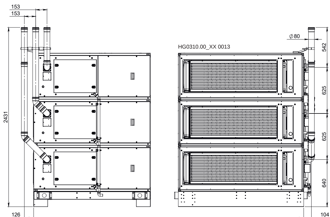
Modello: AH320 (- xxH0) con scarico fumi SINGOLO
