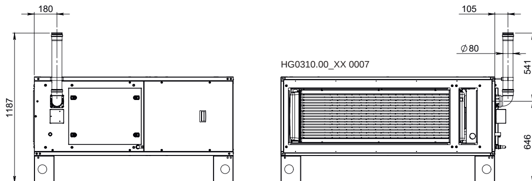
Modello: AH160 / AH210 (- xxH0) con scarico fumi SINGOLO
