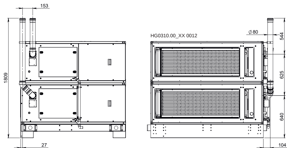
Modello: AH320 (- xxH0) con scarico fumi SINGOLO
