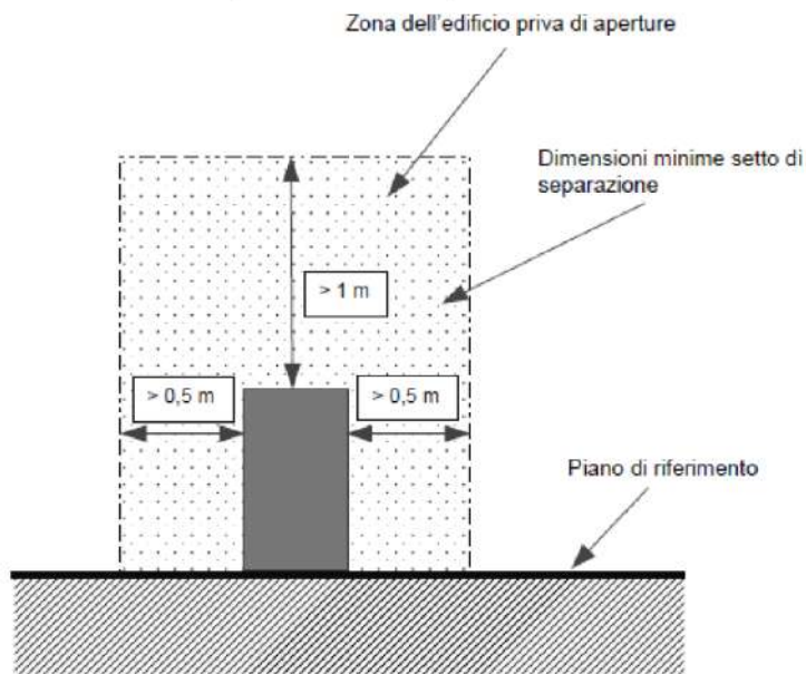
Tavola 4 - installazione all'aperto adiacente a parete
