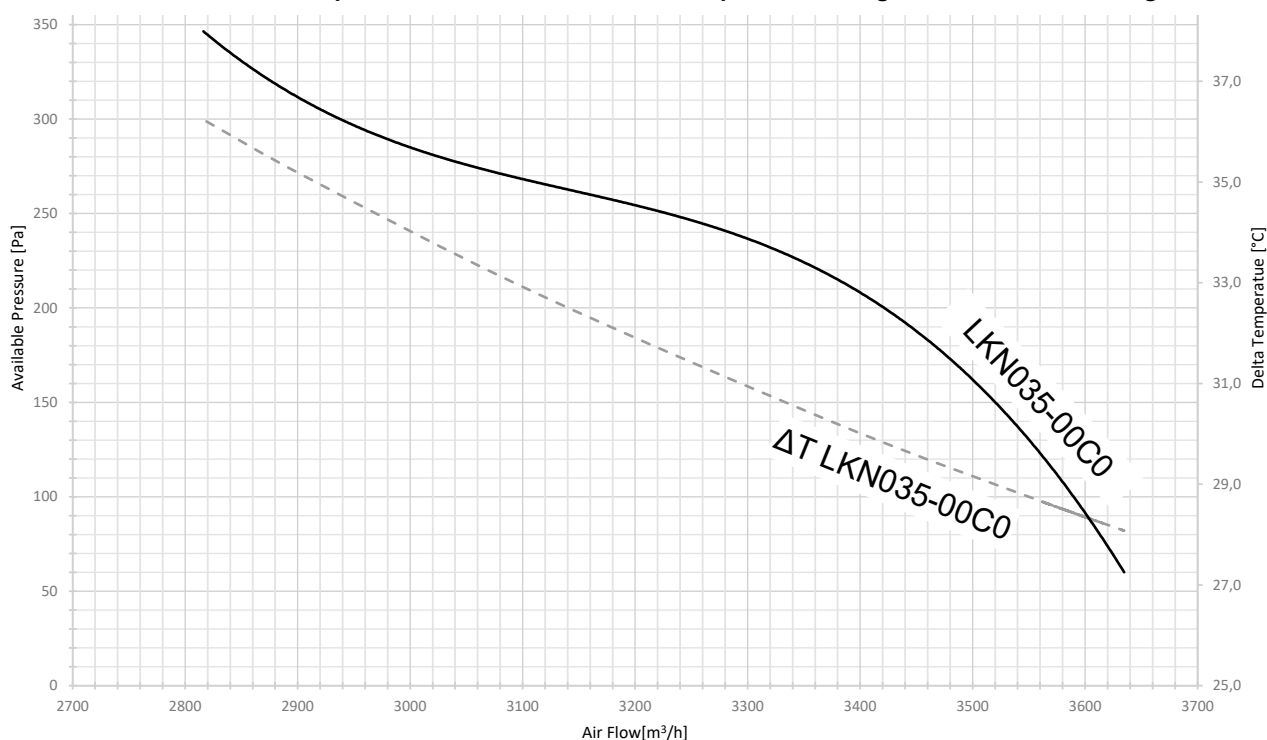
Grafico "Portata aria - perdita di carico - incremento temperatura" dei generatori LKN centrifughi
