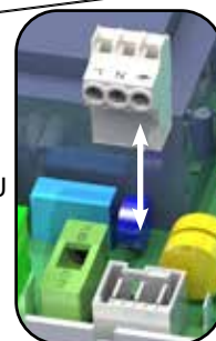
Connettore alimentazione su scheda CPU
