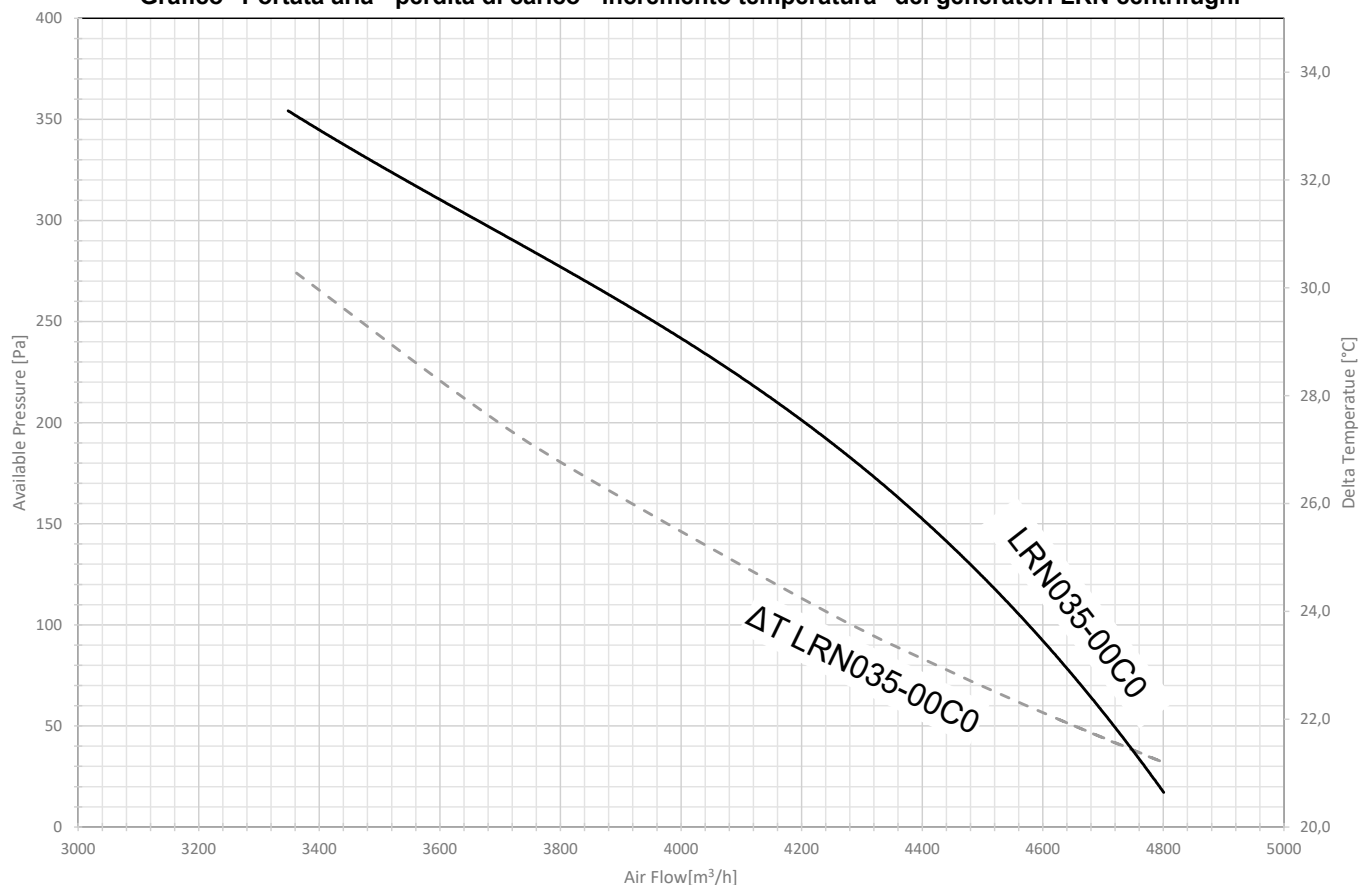
Grafico "Portata aria - perdita di carico - incremento temperatura" dei generatori LRN centrifughi
