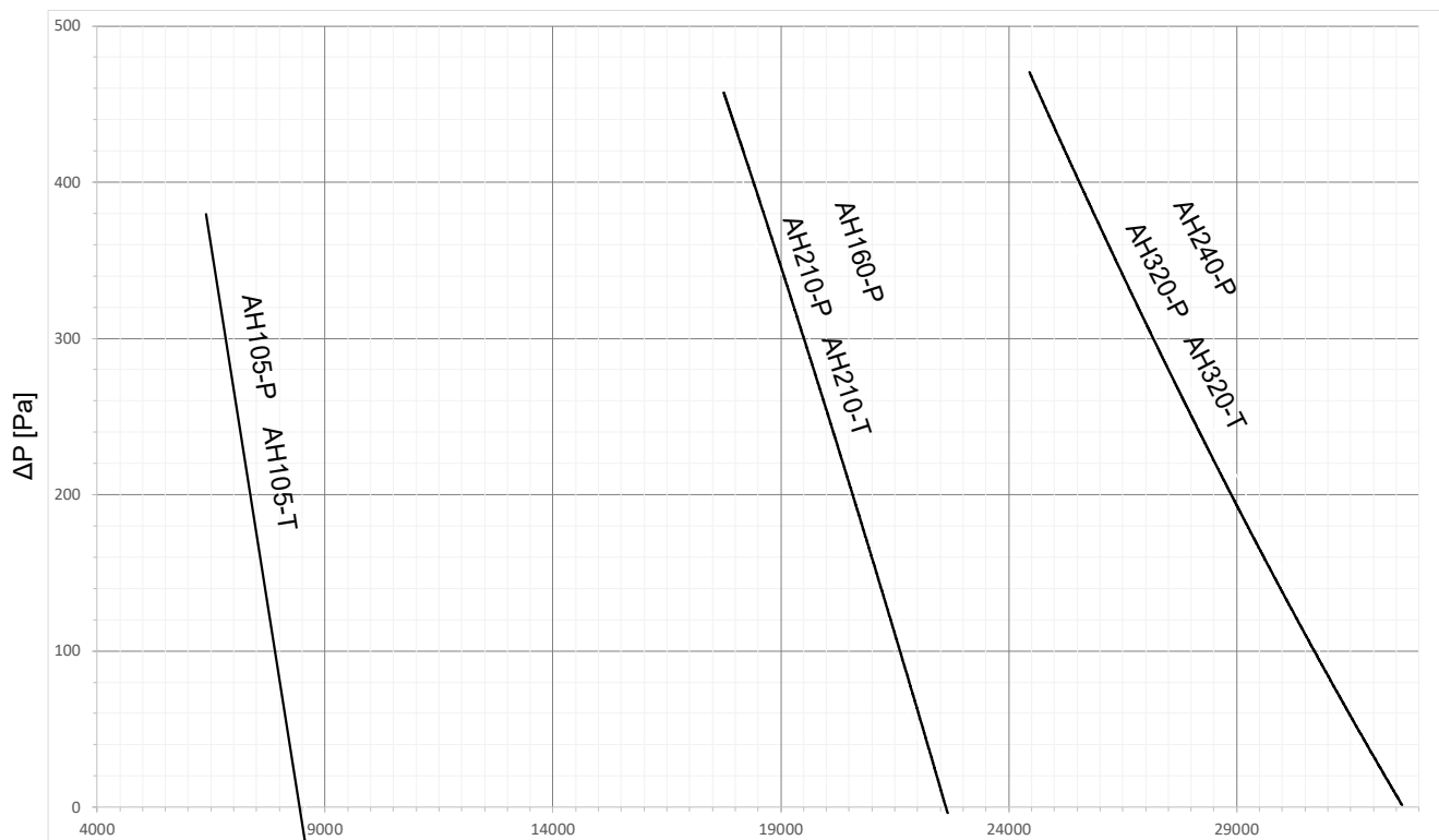
Curva Portata aria
